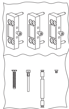
Upevnění závěsu
